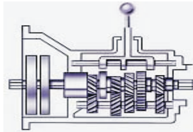
Versnellingsbak
